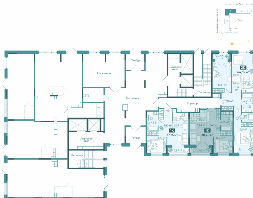
ГП-8, СЕКЦИЯ 3, 1 ЭТАЖ
